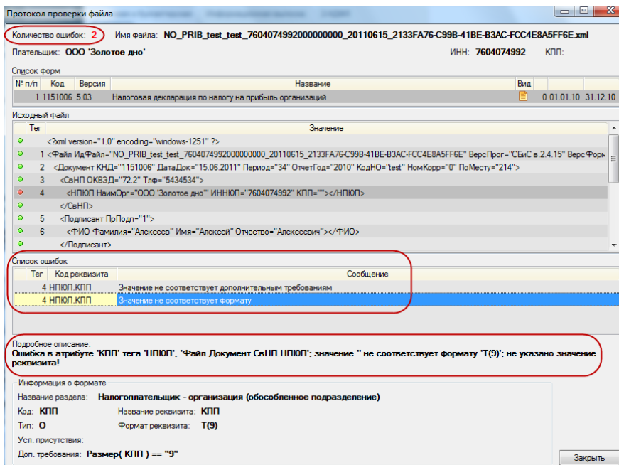
Рис. 12-2 — Фрагмент форматно-логической проверки файла
